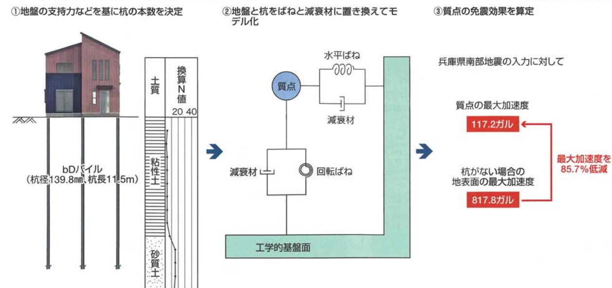
図3-2 計算上は最大加速度を8割以上低減
